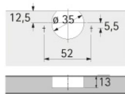
Cotes de perçage TH32 Seleкта Pro 2000
