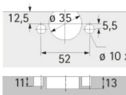
Cotes de perçage TH33 Seleкта Pro 2000
