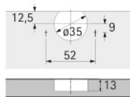
Cotes de perçage TX32/52x9 Seleкта Pro 2000
